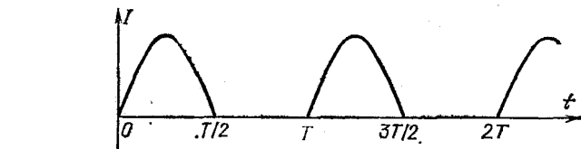
Рис. 316. Форма тока при однополупериодном выпрямлении
