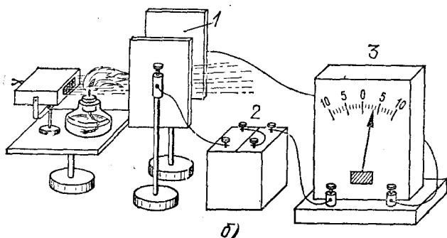
Рис. 148. а) Газ, ионизованный пламенем, проводит электричество. б) Если воздух, ионизованный пламенем, проходит до пластин небольшое расстояние, гальванометр показывает наличие тока, 1 — газовый промежуток, 2 — аккумуляторная батарея, 3 — гальванометр
