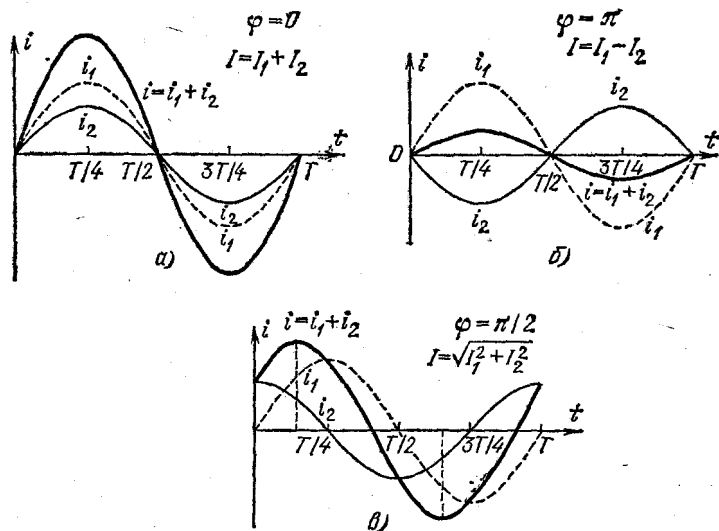
Рис. 303. Сложение двух синусоидальных переменных токов. Складываемые токи: а) совпадают по фазе ( \varphi = 0 ); б) противоположны по фазе, т. е. сдвинуты во времени на половину периода ( \varphi = \pi ); в) сдвинуты во времени на четверть периода ( \varphi = \pi/2 )
