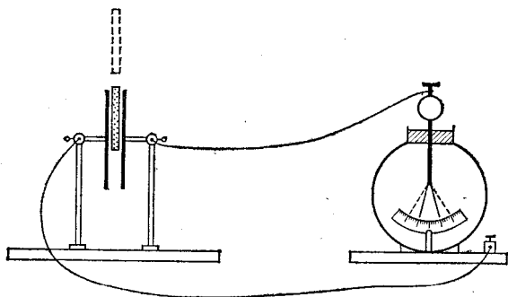
Рис. 63. Емкость конденсатора увеличивается при вдвигании эбонитовой пластинки между его обкладками. Листки электромметра спадают, хотя заряд остается прежним
