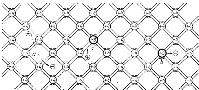
Рис. 185. Схема строения кристалла германия: кружки с цифрой «+4» — атомы германия, кружки с цифрами «+5» и «+3» — внедренные в германий атомы пентавалентного мышьяка и трехвалентного индия
