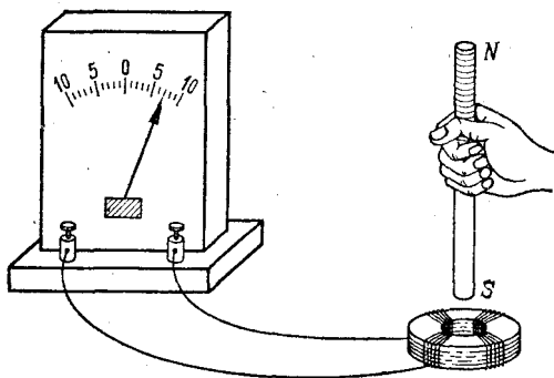
Рис. 253. При относительном перемещении катушки и магнита в катушке возникает индукционный ток: а) катушка надевается на магнит; б) магнит вдвигается в катушку
