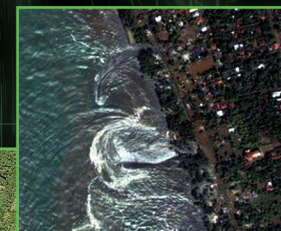
Цунами в прибрежной зоне
